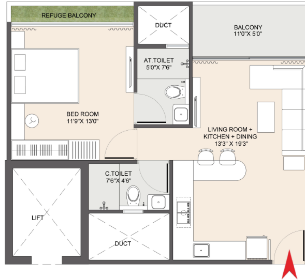
1BHK TYPE 2
